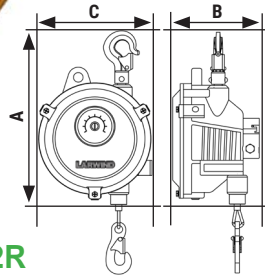
MI-RW0 0,50 - 1,50 Kg
